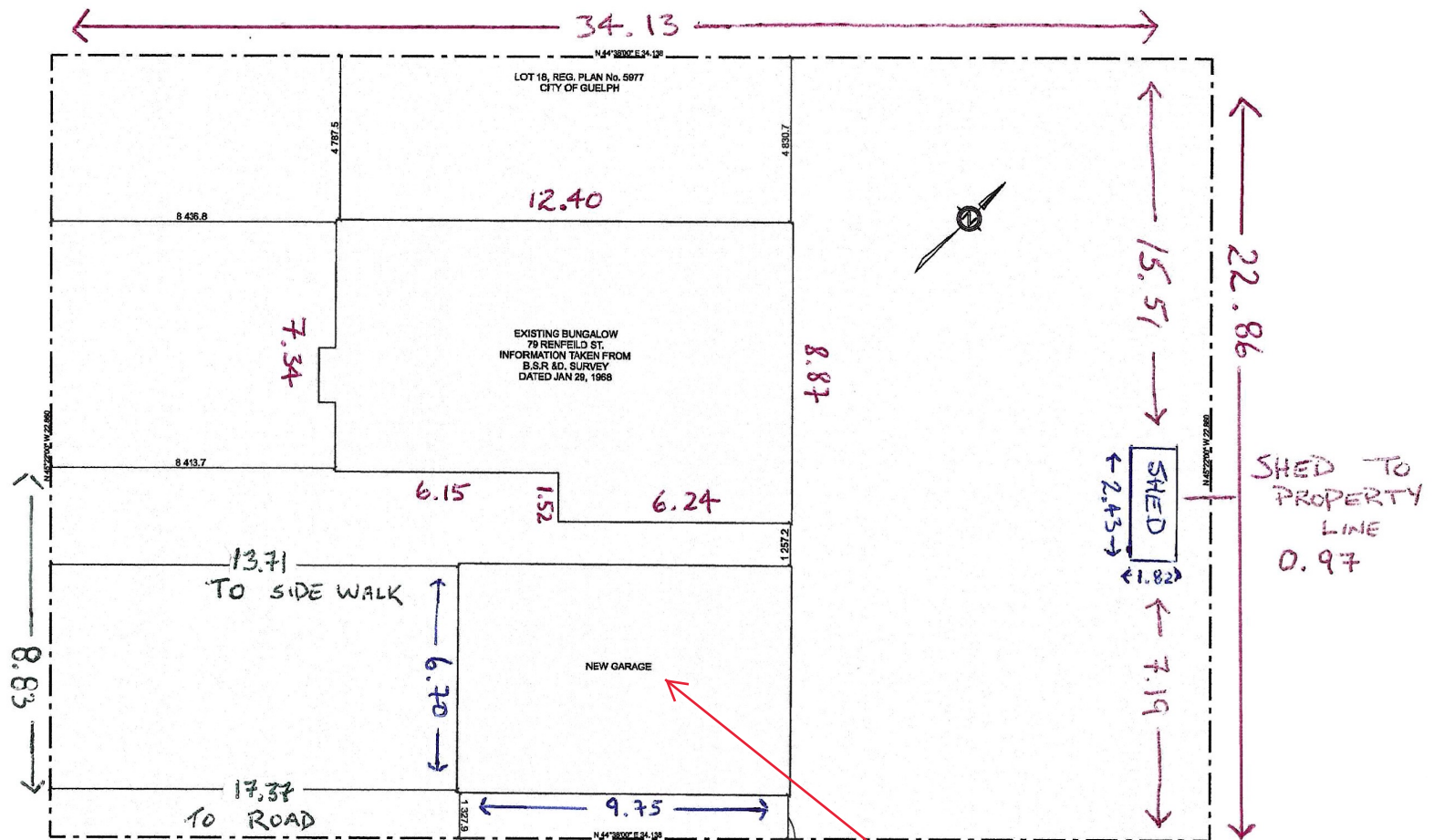
SITE PLAN SCALE: 1:120
