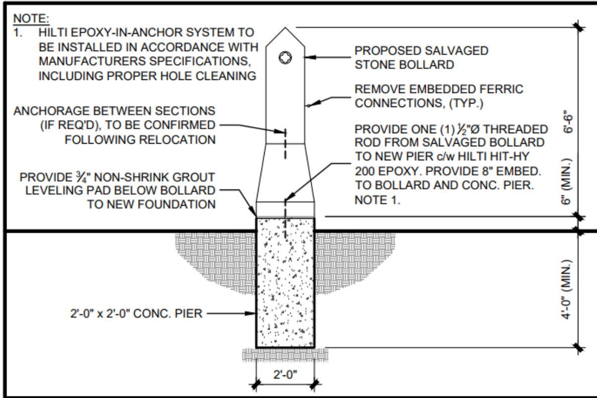
2 S1 SECTION - BOLLARD SCALE: 1/4" = 1'-0"
